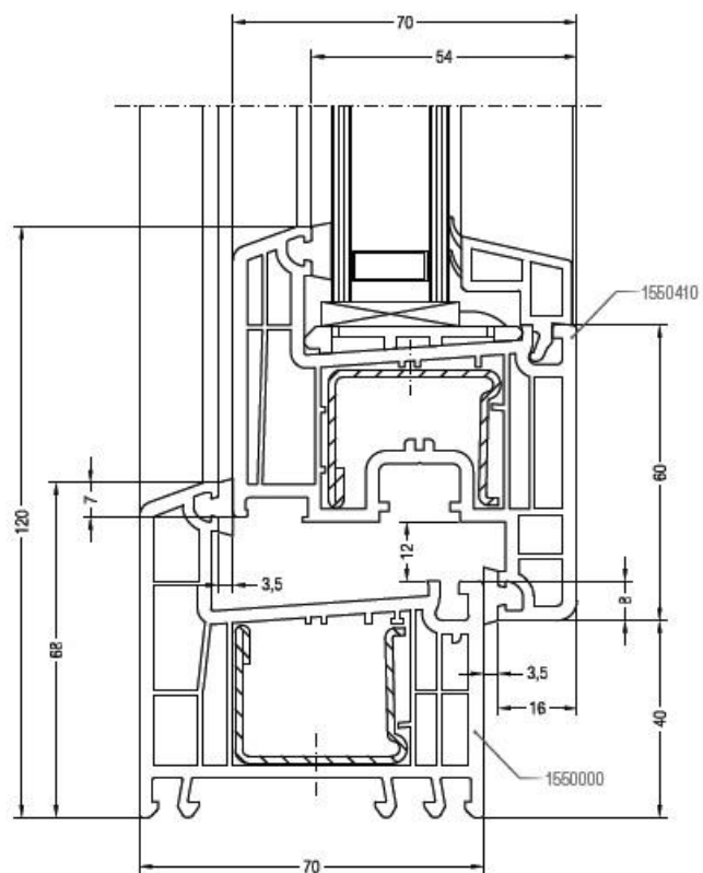
Sezione nodo Brillant 70 anta da 60 mm dritta
